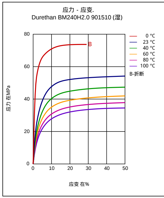
应力 - 应变.
